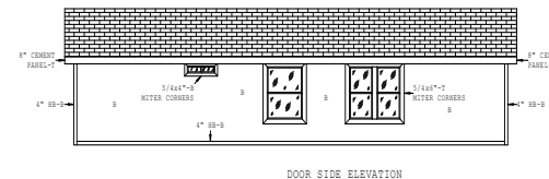
DOOR SIDE ELEVATION
