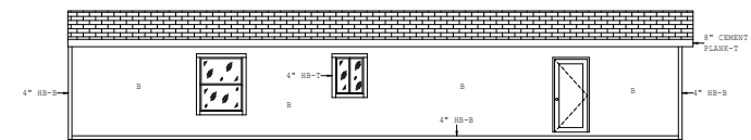
DOOR SIDE ELEVATION
