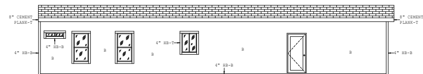
DOOR SIDE ELEVATION
