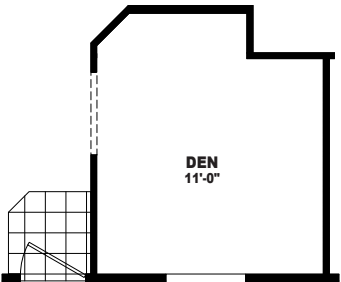
OPTIONAL DEN
